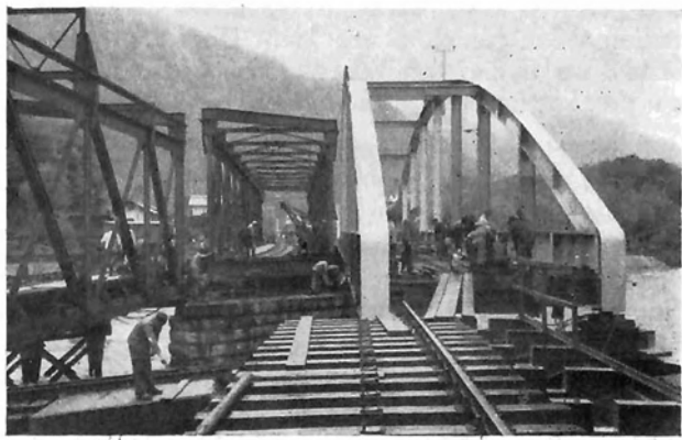
Bild 1c: Auswechslung in der Gleissperre
