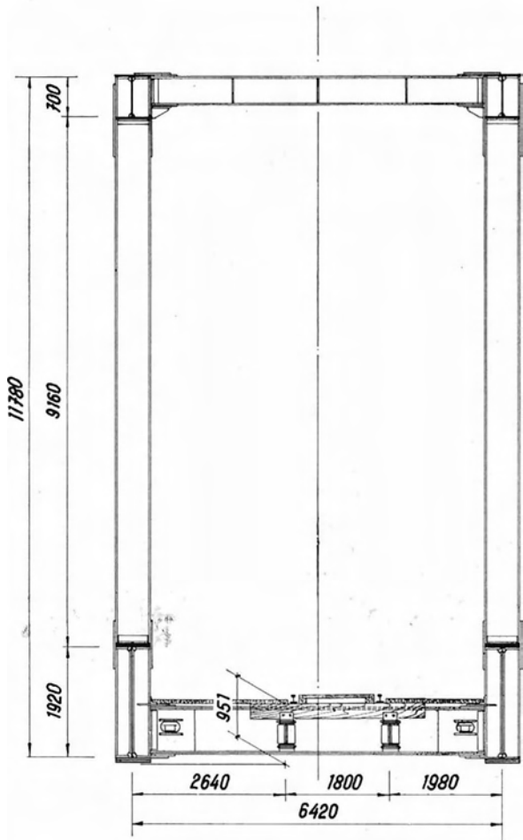
Bild 1b: Querschnitt des Haupttragwerkes
