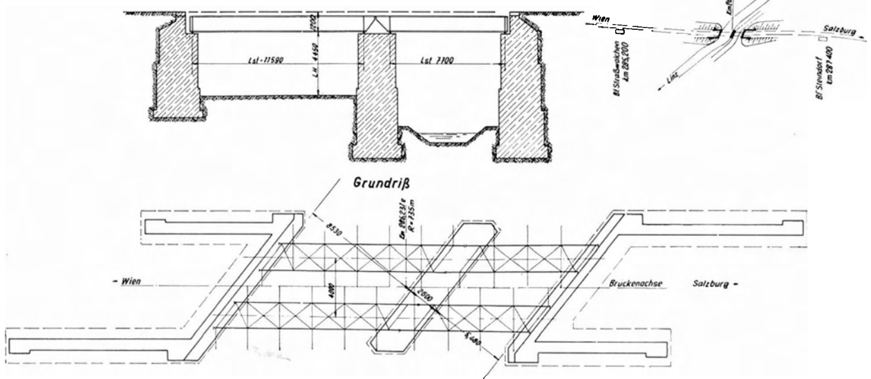
Bild 10: Bundesstraßenunterführung bei Straßwalchen unter der Bahnlinie Wien-Salzburg in km 286,2/3: Alter Bestand (Längenschnitt und Grundriß)
