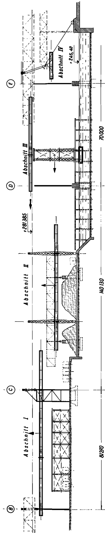
Bild 2: Zweiter Montageabschnitt
