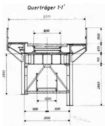
Bild 6a: 2 Querschnitte Fig. 6a: 2 Cross-Sections
