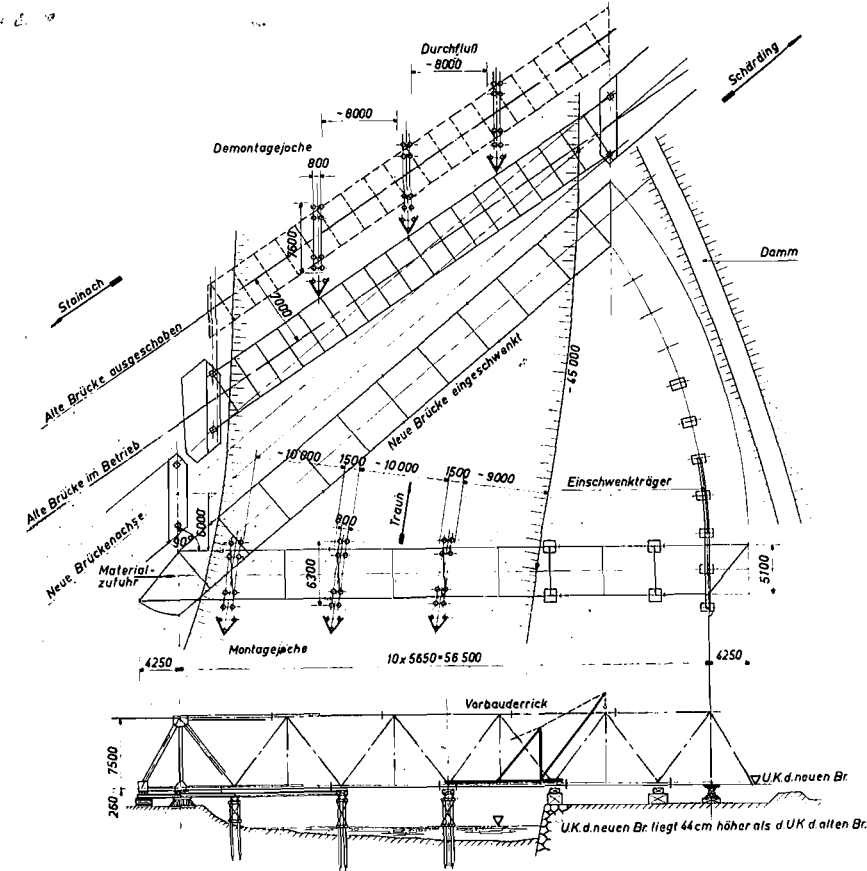
Bild 2b: Montagevorgang
