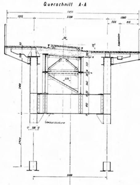
Bild 5a: Querschnitt der neuen Brücke
