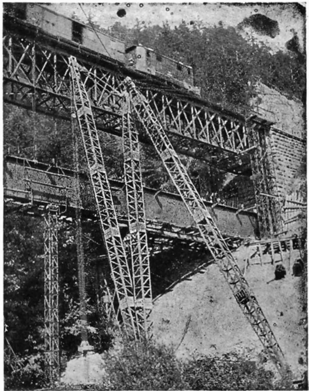
Bild 7: Wallerbachbrücke in km 6,903 der Strecke Stainach-Irdning–Attnang-Puchheim: Montagevorgang
