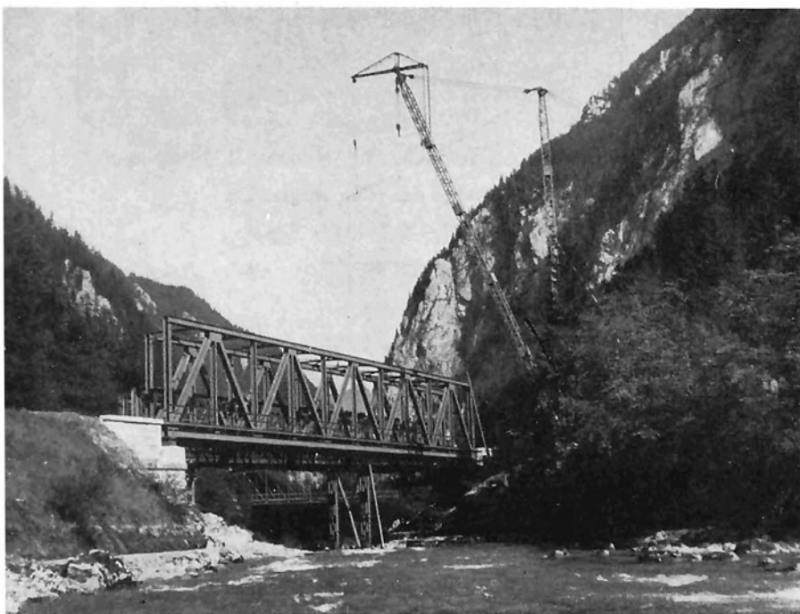
Bild 8a: Ansicht der neuen Brücke. Im Hintergrund altes Tragwerk und dahinter Straßenbrücke
